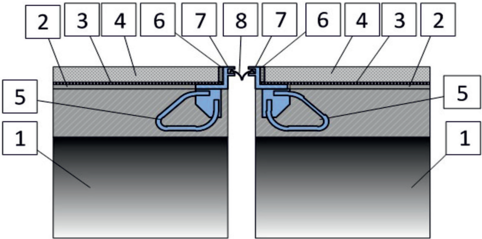
1 – пролетное строение; 2 – выравнивающий слой; 3 – гидроизоляция и защитный слой одежды мостового полотна; 4 – покрытие одежды мостового полотна на слое гидроизоляции; 5 – анкерный элемент; 6 – герметик; 7 – окаймление; 8 – компенсатор
