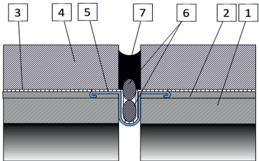
1 – плита проезжей части; 2 – защитный слой; 3 – гидроизоляция; 4 – покрытие проезжей части; 5 – компенсатор; 6 – уплотнитель зазора; 7 – материал заполнения
