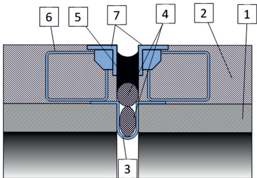
1 – плита проезжей части; 2 – покрытие проезжей части; 3 – компенсатор; 4 – уплотнитель зазора; 5 – материал заполнения; 6 – анкеровка окаймления; 7 – металлическое окаймление
