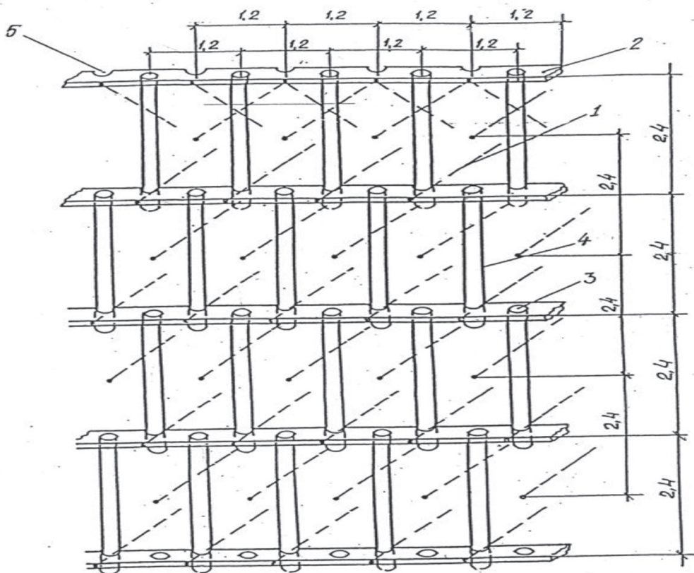
1 – грунтовый нагель с несущим стержнем из АНК; 2 – горизонтальная балка продольного пояса; 3 – кондуктор для устройства стойки; 4 – вертикальная стойка; 5 – стыковочный паз
