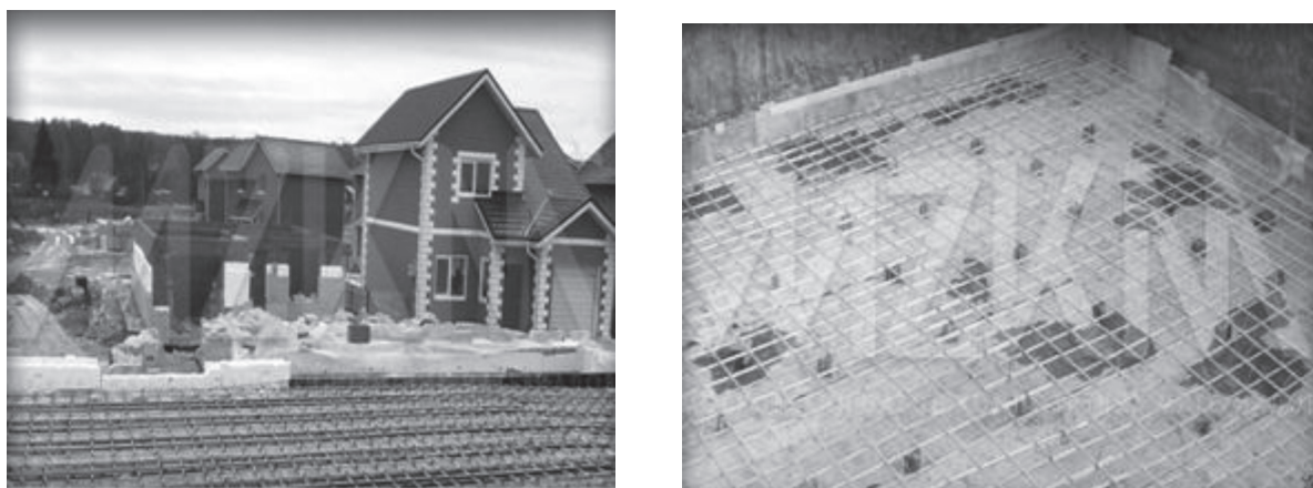
Рисунок 8.3 – Применение АНК для армирования фундаментной плиты 1)
