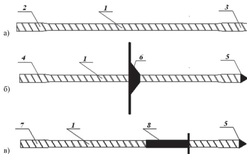
1 – стержень из АНК-С; 2 – анкерное уширение диаметром 5,6 мм; 3 – уширение с заточкой; 4 – анкерное уширение диаметром 7,7 мм; 5 – пластмассовый наконечник; 6 – распорная шайба; 7 – анкерное уширение диаметром 10,5 мм; 8 – технологический ограничитель
