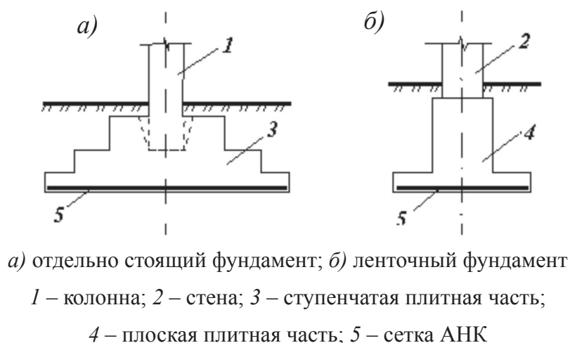
Рисунок 8.2 – Схема армирования фундаментной плиты
