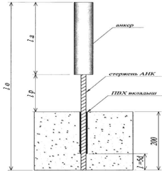
Рисунок Г.2 – Схема установки стержня в бетон
