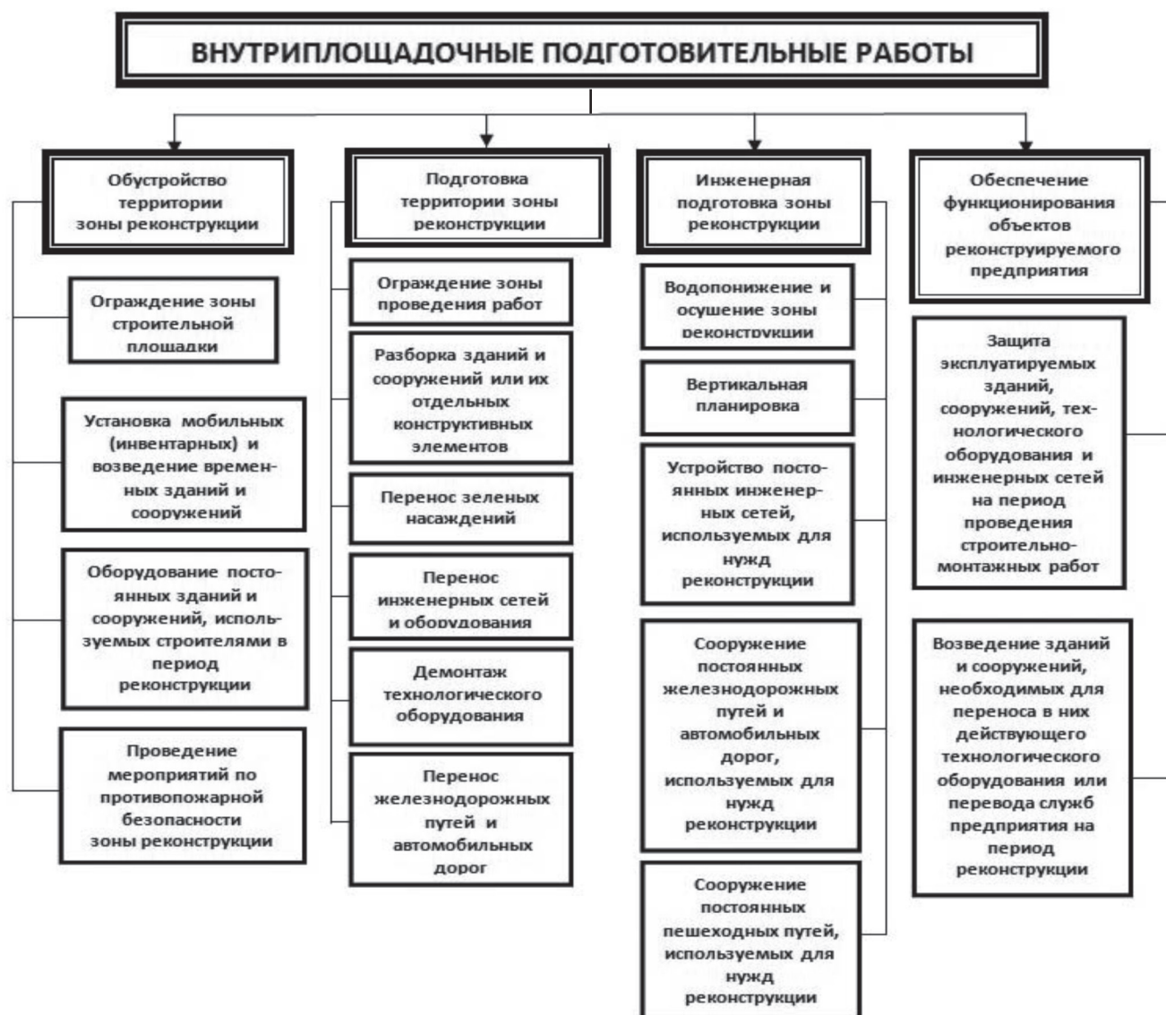
Рисунок 7 – Схема внутриплощадочных подготовительных работ
