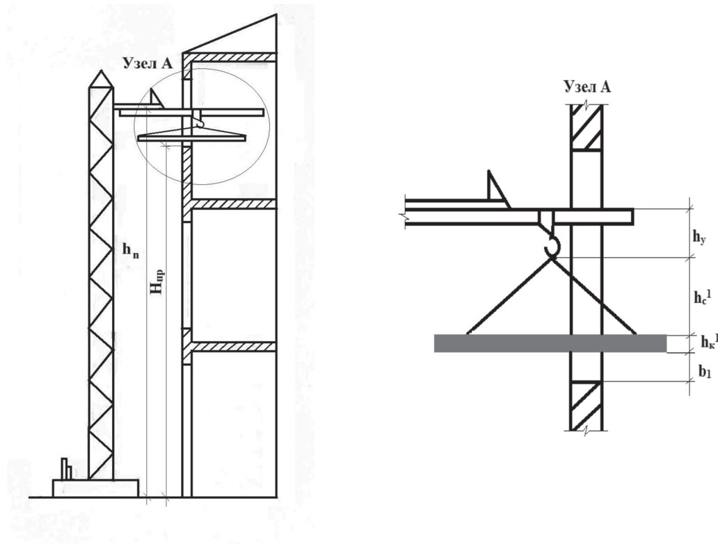
Рисунок 4 – Монтаж конструкций через проемы здания
