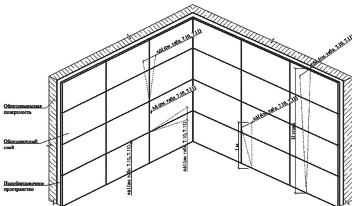
Рисунок 15 – Контролируемые параметры выполненной конструкции облицовочного слоя
