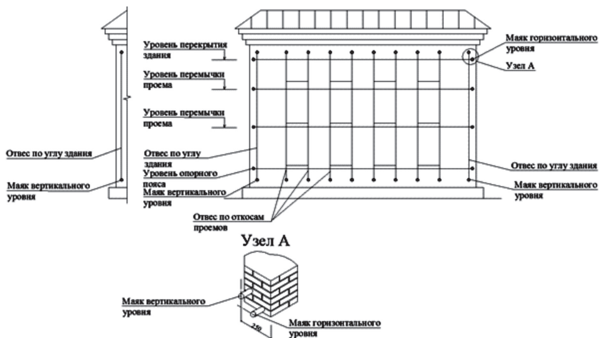
Рисунок 7 – Схема расположения отвесов и горизонтальных шнуров
