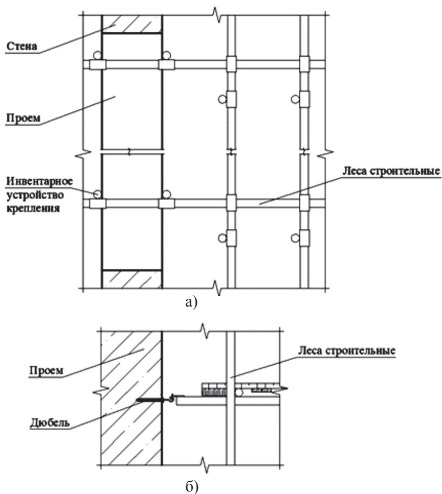
Рисунок 6 – Вариант крепления лесов строительных
