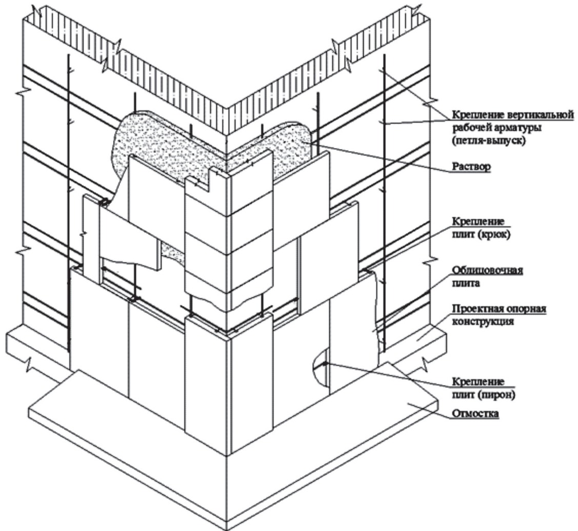
Рисунок 11.2 – Схема крепления облицовочных плит на угловом участке по типу 3
