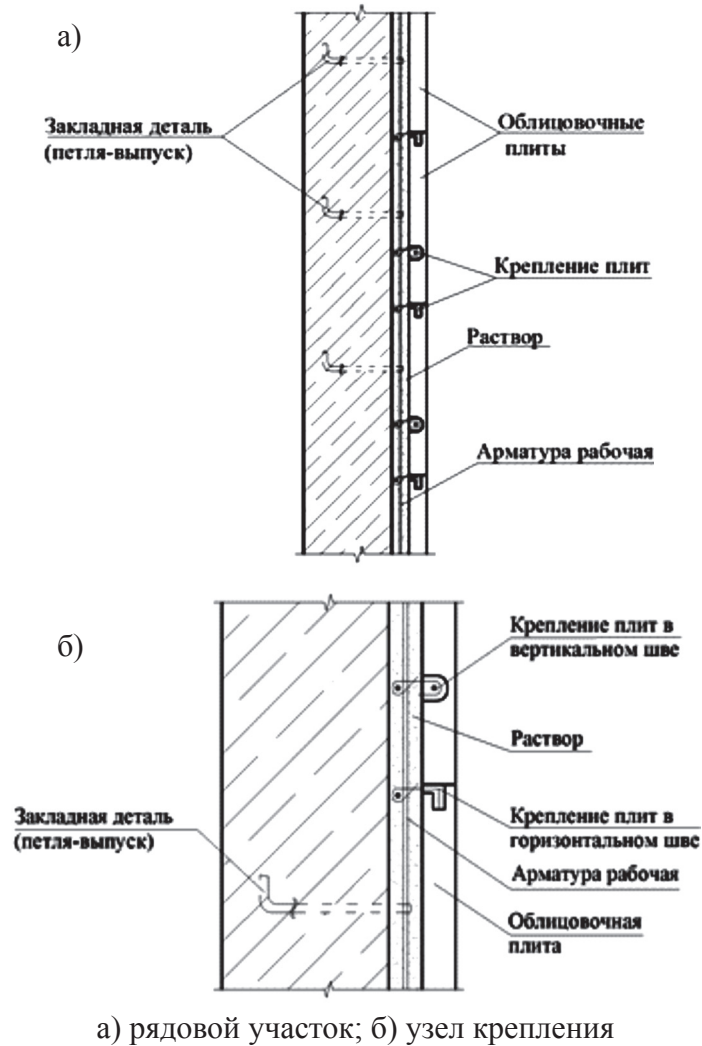
Рисунок 3 – Схема устройства облицовочного слоя (тип 3)
