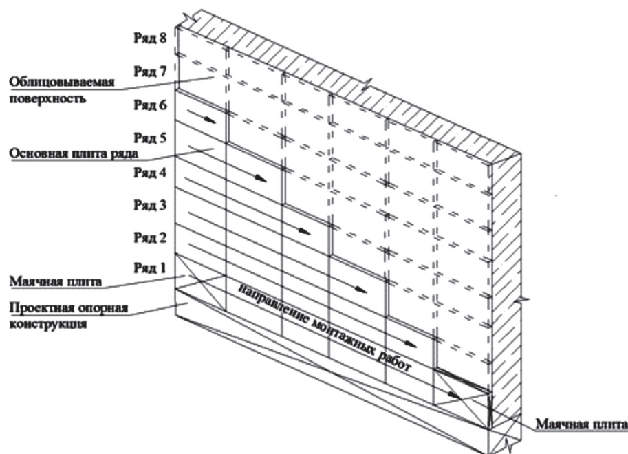
Рисунок 14 – Порядок монтажа облицовочной плитки (тип 4)
