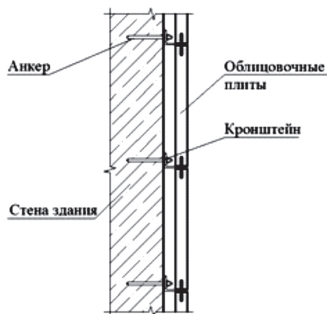
Рисунок 1 – Схема устройства облицовочного слоя (тип 1)
