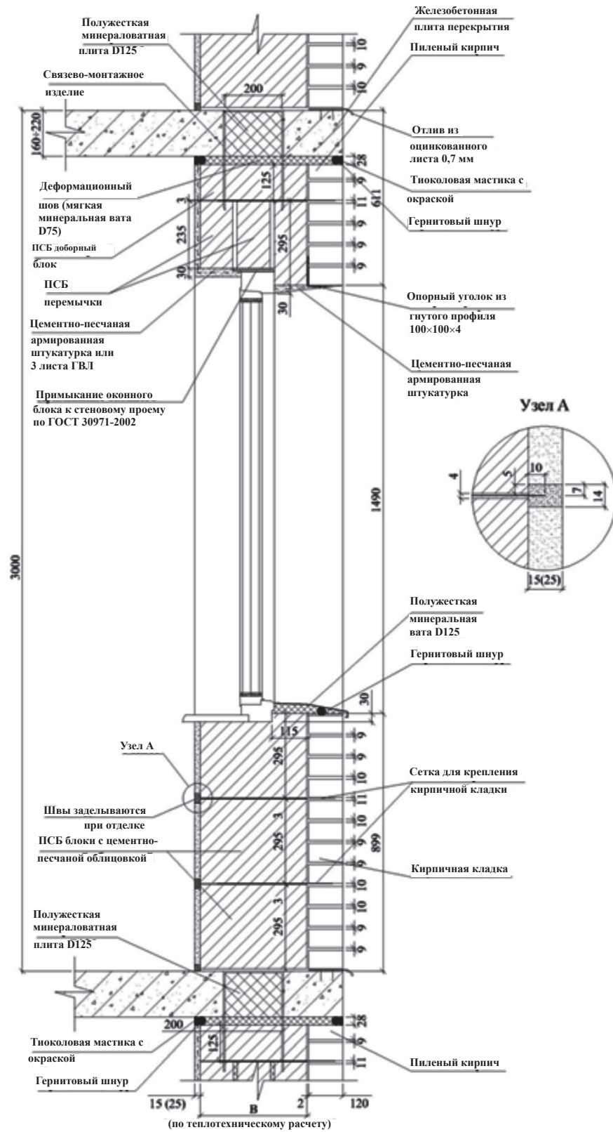
Рисунок 6.6 – Ненесущая стена из ПСБ блоков с заводской цементно-песчаной облицовкой и наружной кирпичной облицовкой толщиной в 0,5 кирпича.
