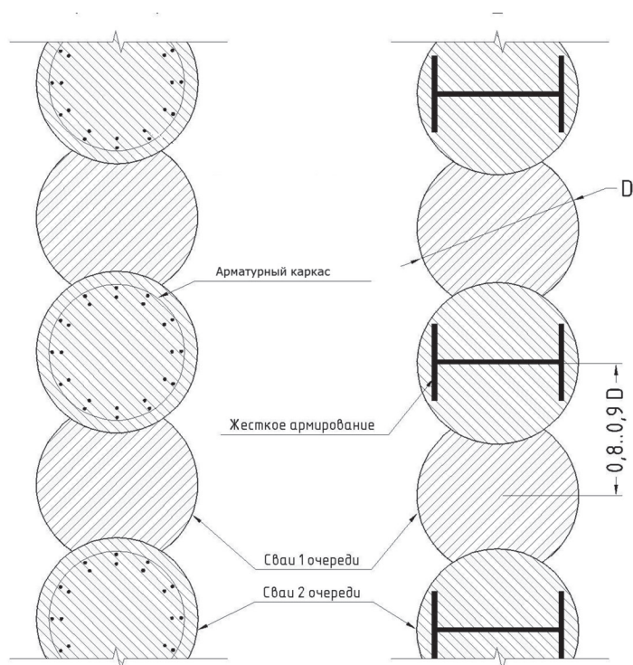
Рисунок 1 – Буросекущие сваи, схема армирования
