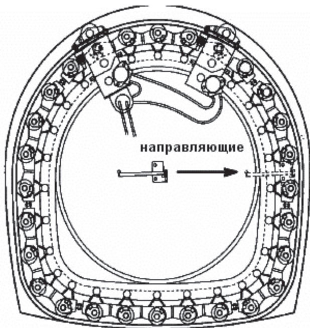
Рисунок 14 – Монтаж направляющей
